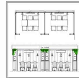
2 CUBICALS
